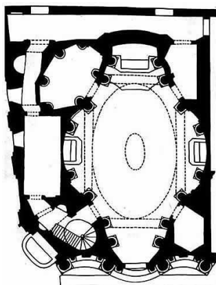
San Lorenzo | San Carlo alle Quattro Fontane, Borromini | Bernini, Sant'Andrea al Quirinale
